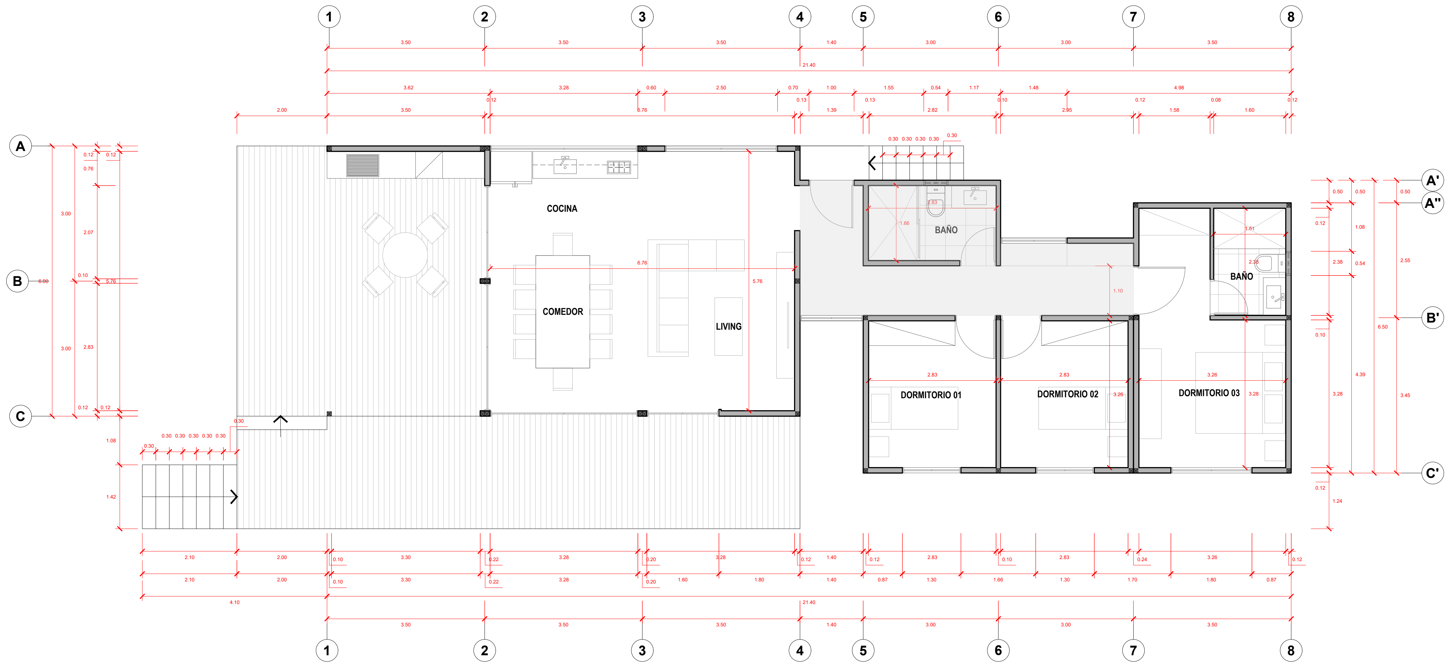
PLANO DE DISTRIBUCION ESC: 1/50
