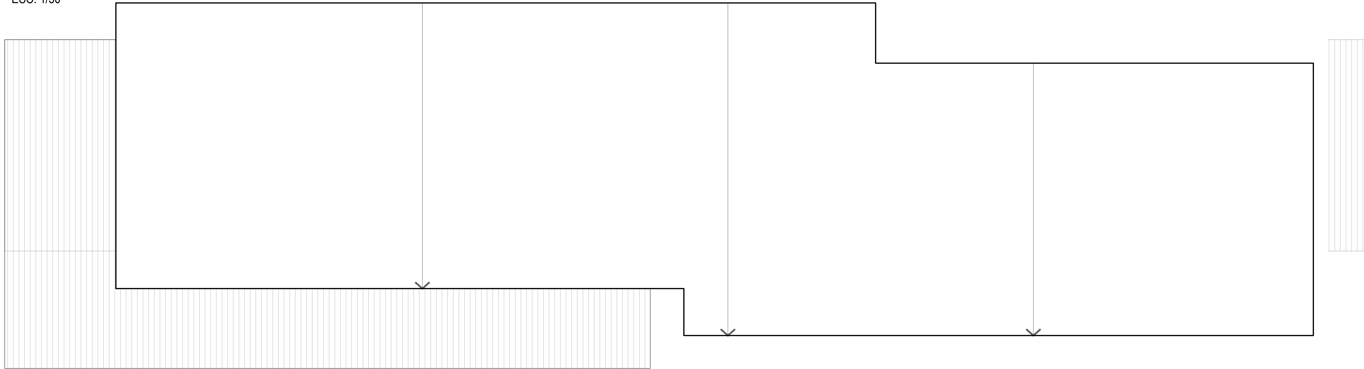
PLANO DE DISTRIBUCION ESC: 1/50
