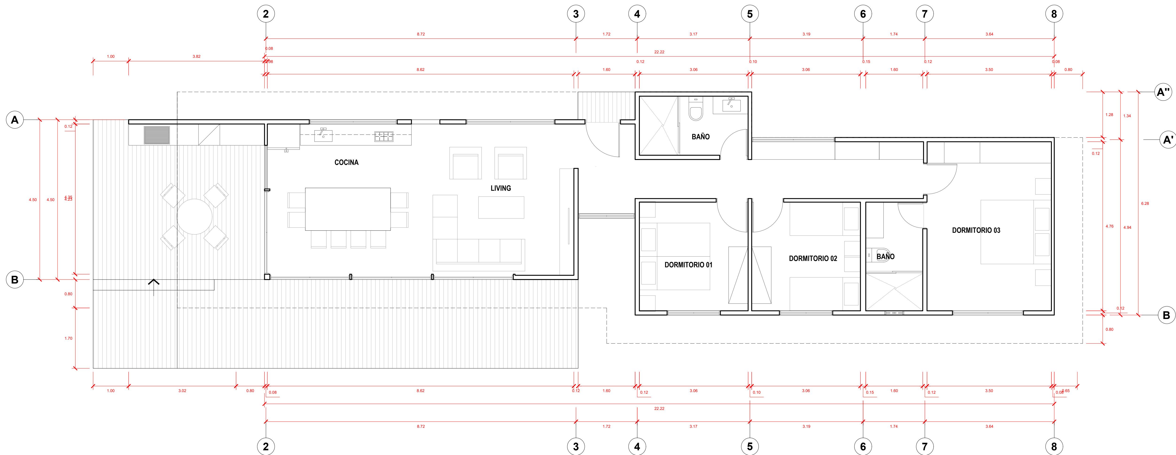
PLANO DE DISTRIBUCION ESC: 1/50
