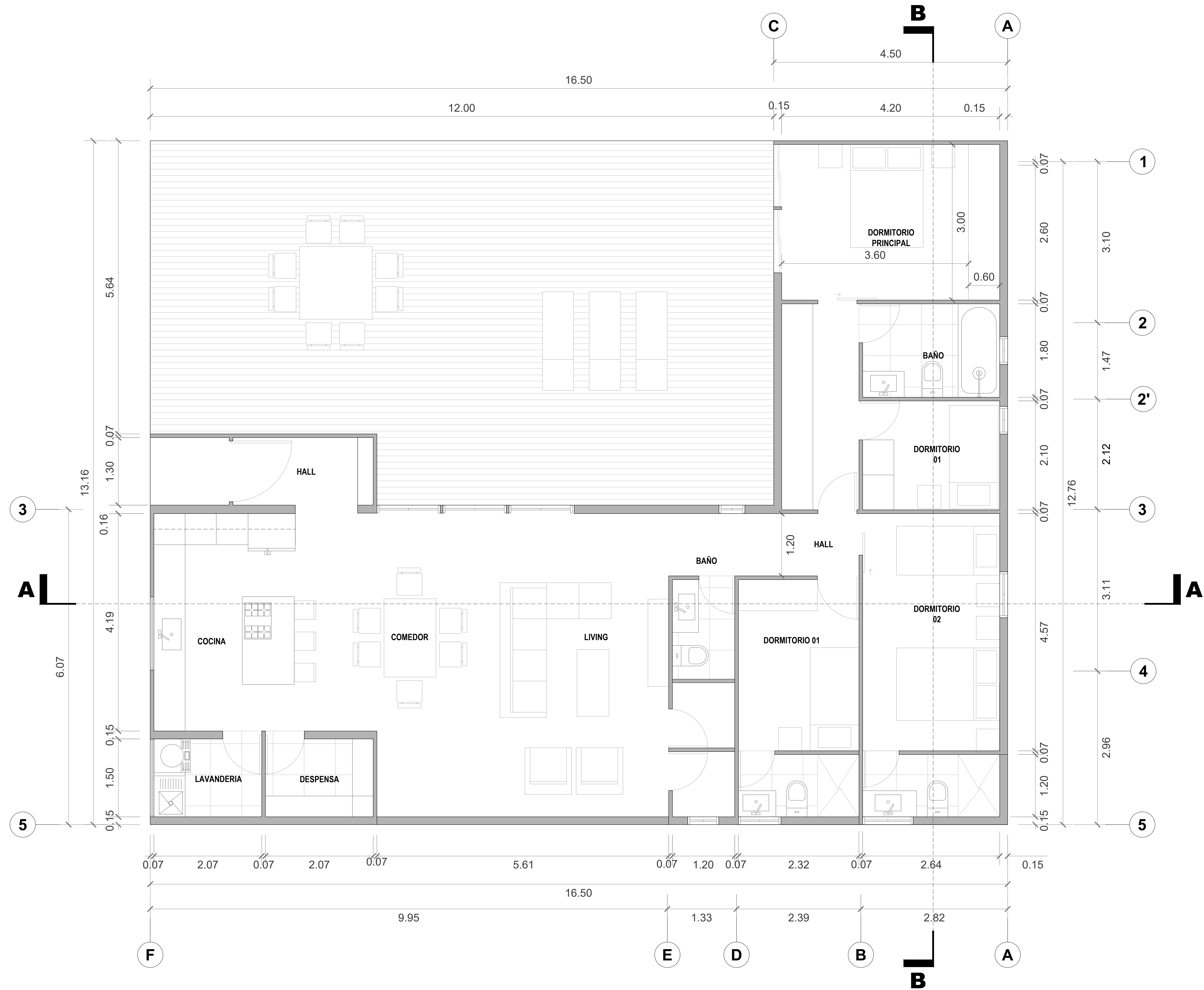
PLANTA DE ARQUITECTURA ESC: 1/75
